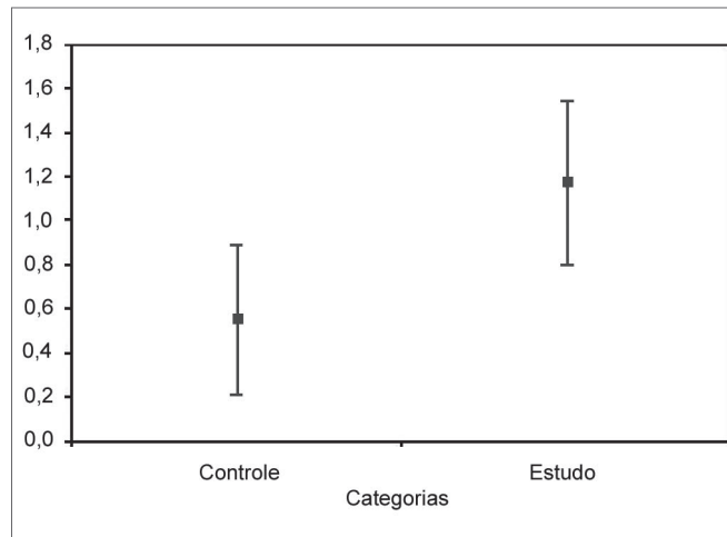
Gráfico 2. T-independente
