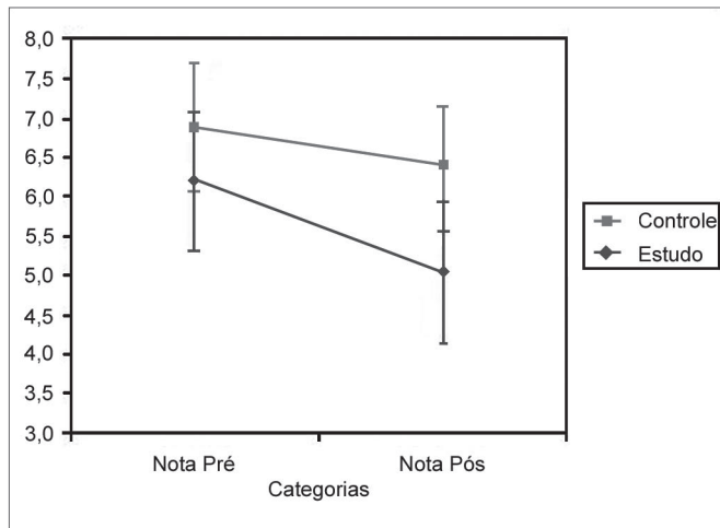
Gráfico 1. Anova.
